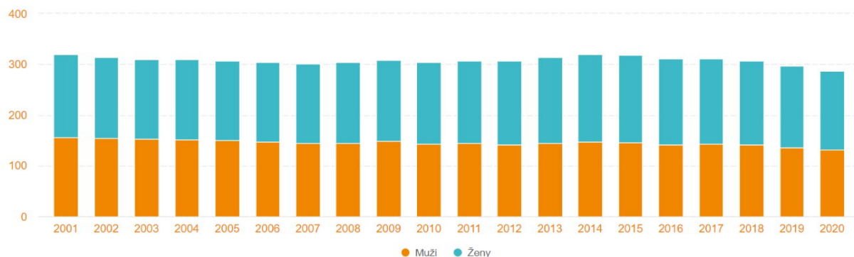
Graf 1 - Zastúpenie mužov a žien na celkovom počte obyvateľov obce Hrišovce (vývoj v období rokov 2001-2020)
