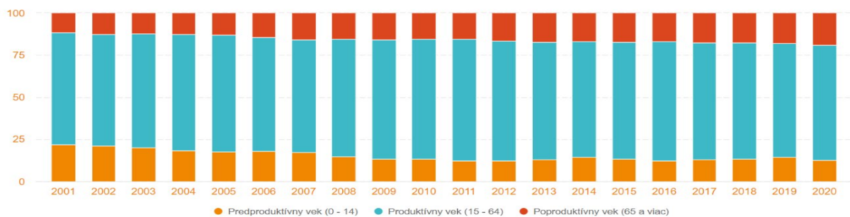
Graf 3 – Ekonomická štruktúra obyvateľov z hľadiska veku v obci Hrišovce od r. 2001 (v %)
